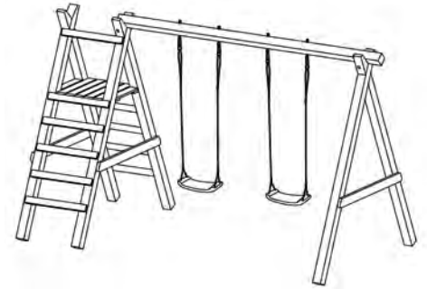
PREMIUM-SCHAUKEL LAURA in Lärche naturbelassen, mit Leitern, Podest, 2 Schaukel- sitzen, XXL-Schaukelbalken 300 cm lang, ohne Rutsche, Gesamtabmessung ca. L 370 x T 190 x H 220 cm 349,99 EUR 8112292
