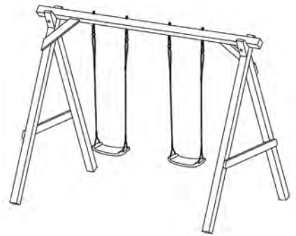
PREMIUM-SCHAUKEL LARA in Lärche naturbelassen, mit Schaukelsitzen, XXL- Schaukelbalken 300cm lang, Gesamtabmessung ca. L 300 x T 190 x H 220 cm 249,99 EUR 8112309
