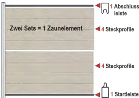
WPC in sand mit Pfosten, Anschlüssen, Designleisten in anthrazit
